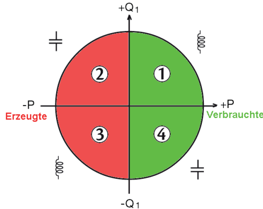
Abbildung 123: 4-Quadranten-Diagramm
