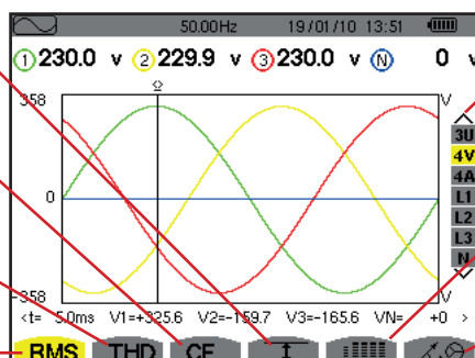
Modus Wellenformen
