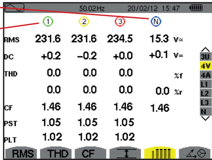
Abbildung 79: Bildschirm zur gleichzeitigen Anzeige bei 4V
