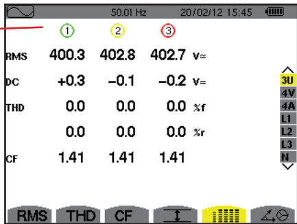
Abbildung 78: Bildschirm zur gleichzeitigen Anzeige bei 3U
