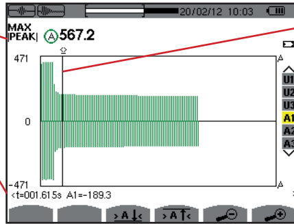
Abbildung 50: Bildschirm zur PEAK -Anzeige bei A1 für dreiphasigen Anschluss ohne Neutralleiter
